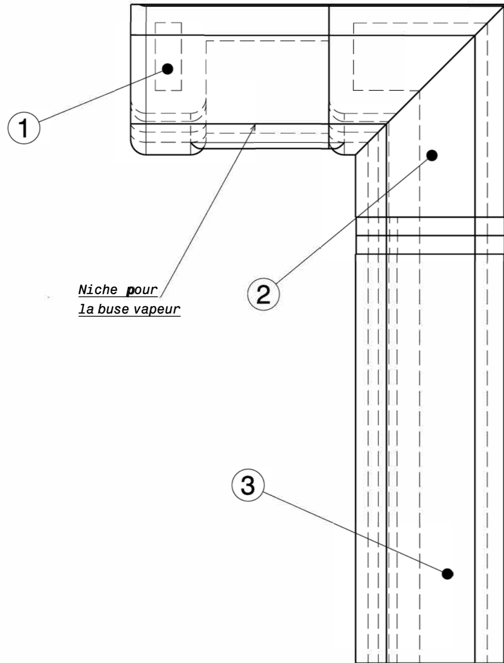
Vue de face Echelle: 1:12
