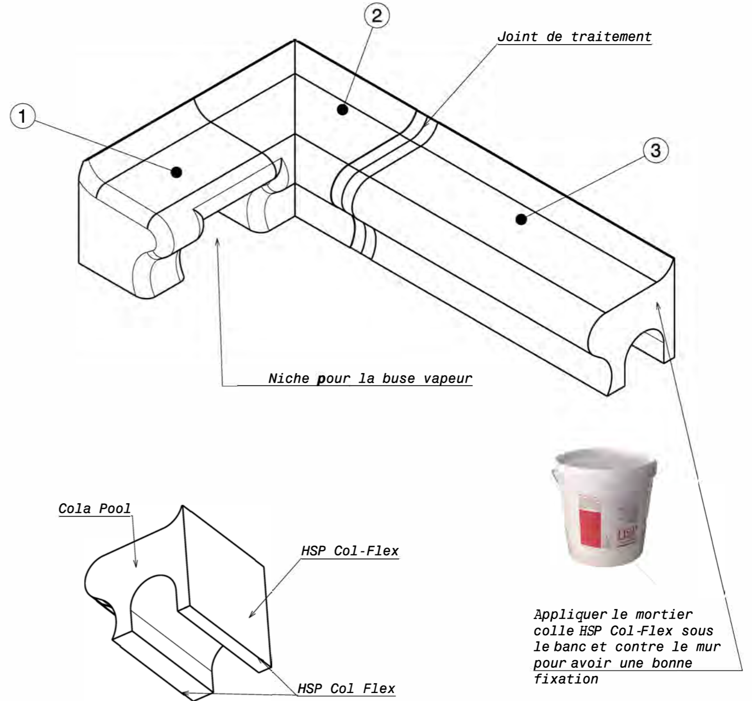
Vue isométrique Echelle: 1:25
